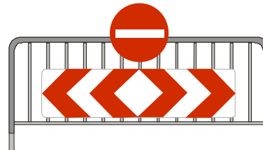
C,1a + E,24ba
