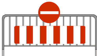
C,1a + E,24aa
